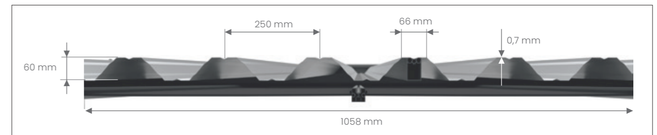
Przekrój blachy trapezowej T60P | Cross-section through trapezoidal sheet T60P (mm)
